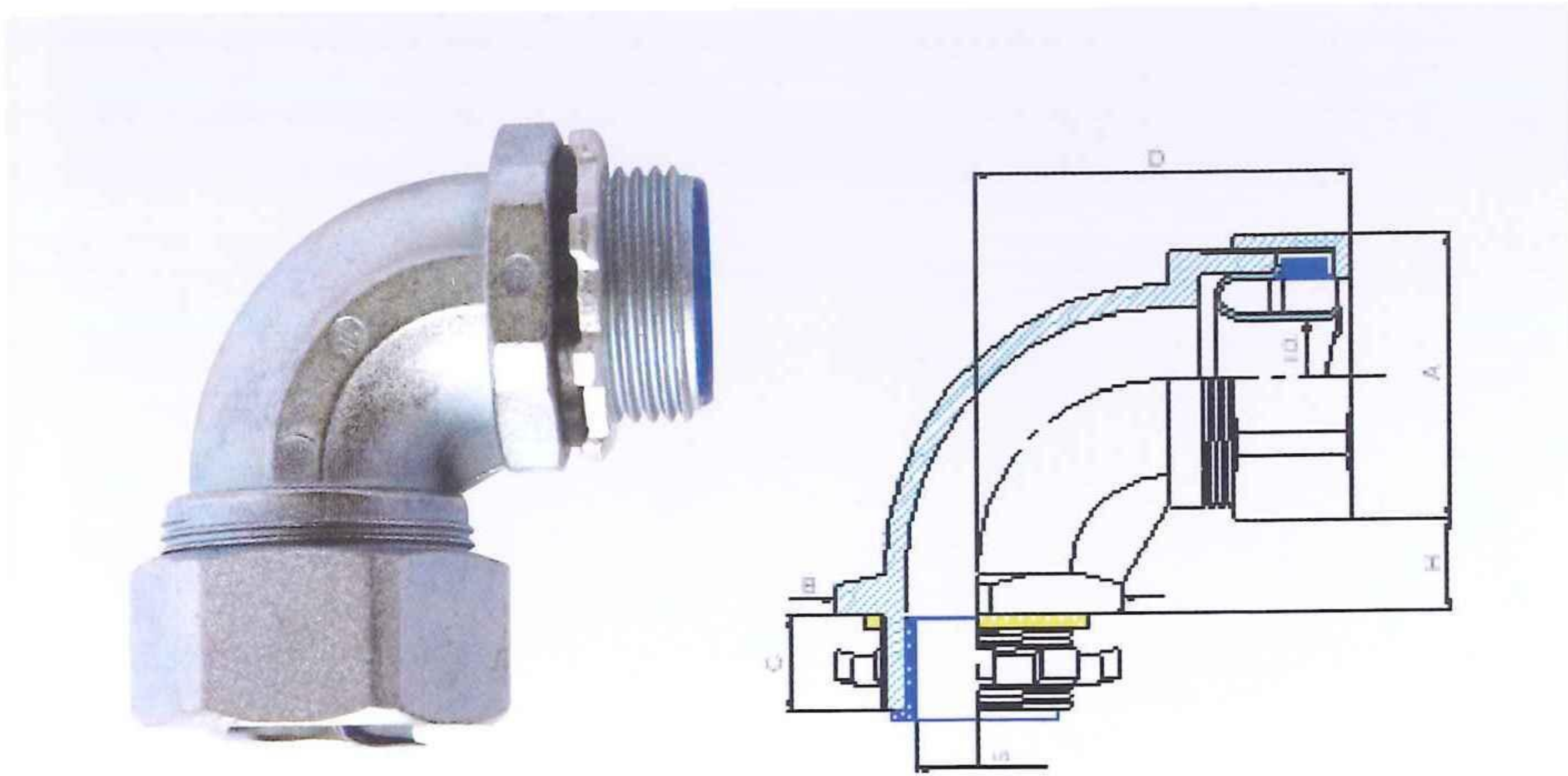
TYPE ZGLM (外螺紋接頭90°)
